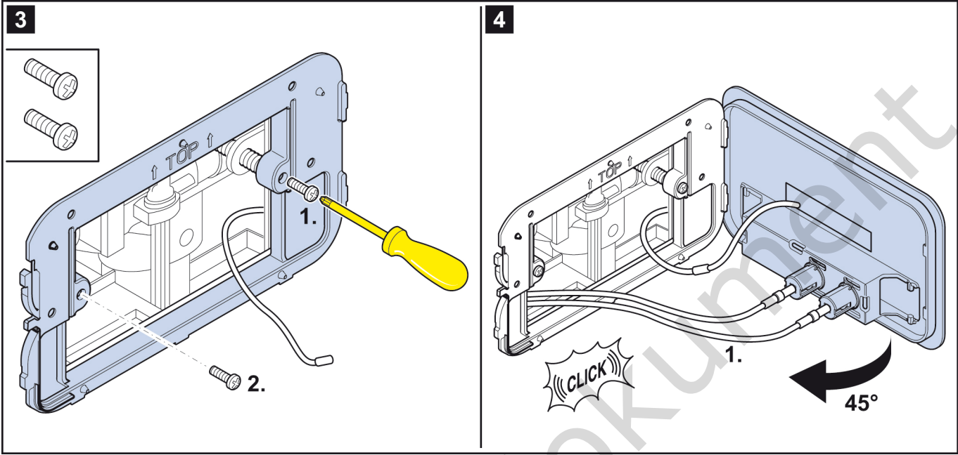
3. Drückerplatte einbauen, siehe Bild 5.
