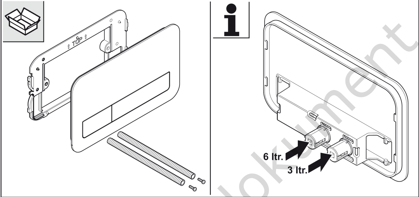
1. Fixer la plaque support avec les vis.
