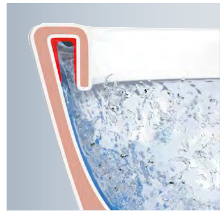
WC con brida.
