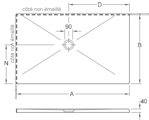
SUBWAY INFINITY MONTAGE EN ANGLE, À GAUCHE CONTRE LE MUR
