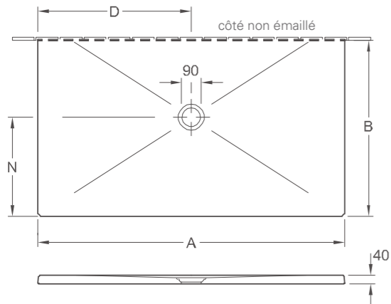
SUBWAY INFINITY CÔTÉ LONG DÉCOUPÉ CONTRE LE MUR
