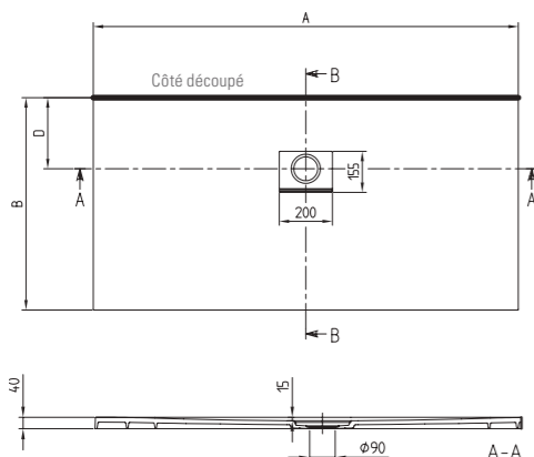
SQUARO INFINITY CÔTÉ LONG DÉCOUPÉ, CONTRE LE MUR
