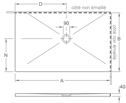
SUBWAY INFINITY MONTAGE EN ANGLE, À DROITE CONTRE LE MUR
