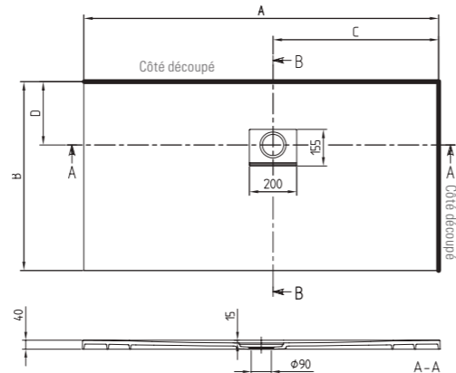
SQUARO INFINITY MONTAGE EN ANGLE, À DROITE CONTRE LE MUR
