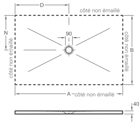
SUBWAY INFINITY UNIQUEMENT POUR ENCASTREMENT À FLEUR
