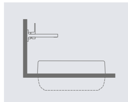
Einbauwaschtisch für Wandauslauf-Armatur.
